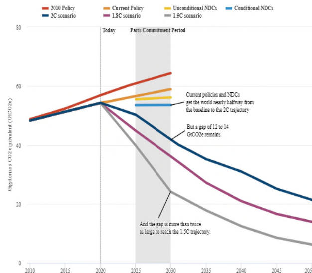
Afbeelding 4: Uitstootscenario's en het gat tussen huidige beleid (oranje) en beleid noodzakelijk om 1,5 graad te bereiken (grijs). Carbon Brief
